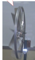
簡易風力 発電機
